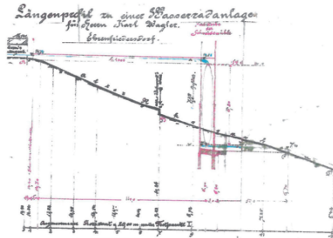
Längsprofil Wasserradanlage
