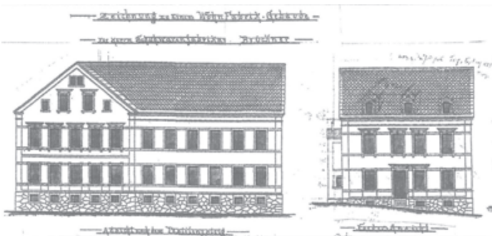
1895 – Neubau Wohn- und Fabrikgebäude Schillerstraße 36
