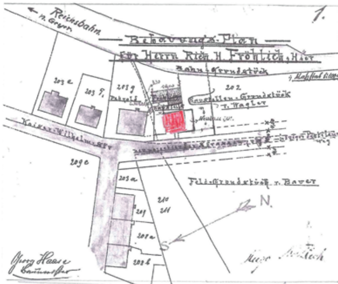
1912 - Lageplan Hugo Fröhlich (Straßenbau bis Fuchshübelstraße fertig - von da ab noch Pestilenzsteig!)
