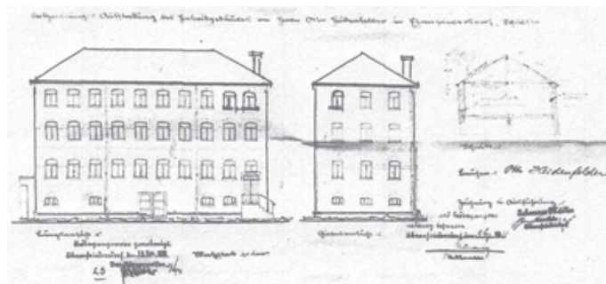
1938 – Aufstockung des Fabrikgebäudes Otto Heidenfelder – Schulstraße 2
