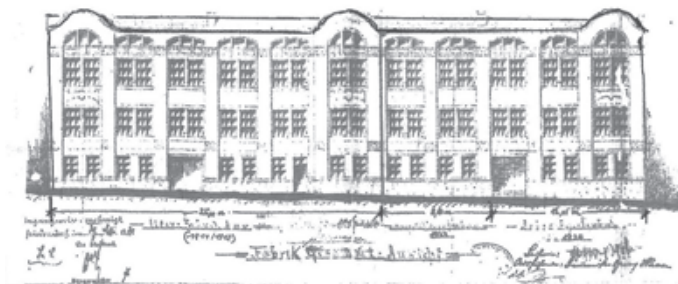
1924 – Gesamtansicht Fabrik, bestehende aus drei Bauabschnitten
