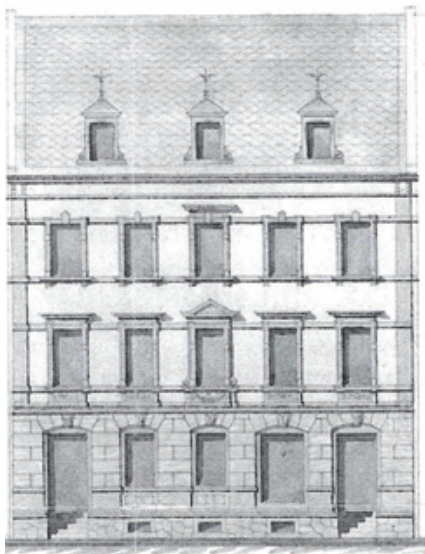
Ansicht Zeichnung Annaberger Str. 8 (1896)
