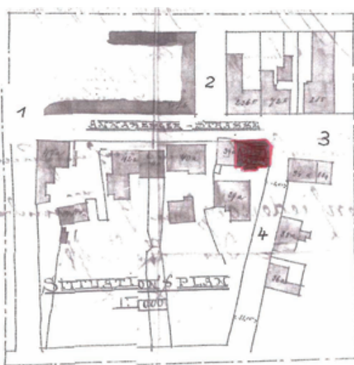
Lageplan Neueinordnung Annaberger Str. 14 (1-4 wie Bild 1)
